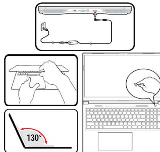
Figure 1 - Ouvrir le couvercle/ordinateur avec un adaptateur AC/DC branché
