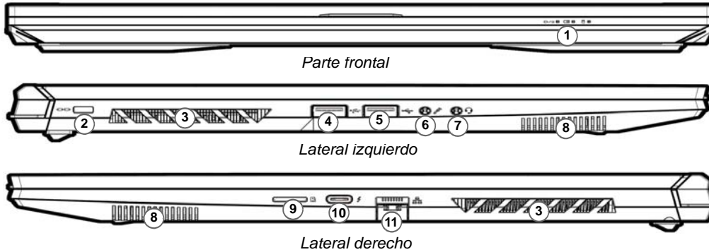
Figura 4 Vistas frontal, izquierda y derecha (Modelo B)
