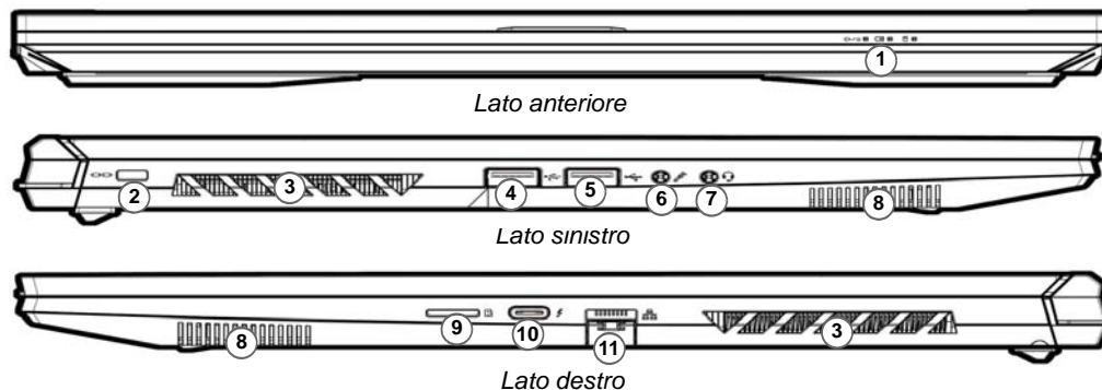
Figura 4 Vista anteriore, sinistra e destra (Modello B)
