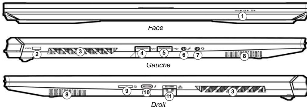
Figure 4 Vues de face, gauche et droite (Modèle B)
