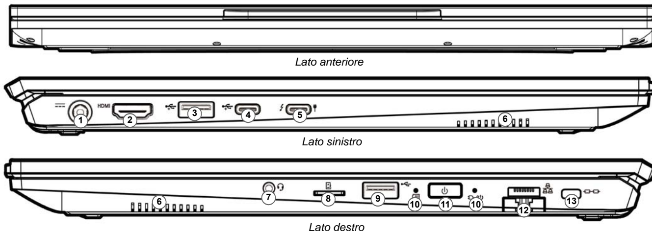
Figura 5 - Vista anteriore, sinistra e destra (Modello B)
