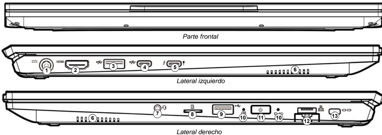
Figura 5 - Vistas frontal, izquierda y derecha (Modelo B)
