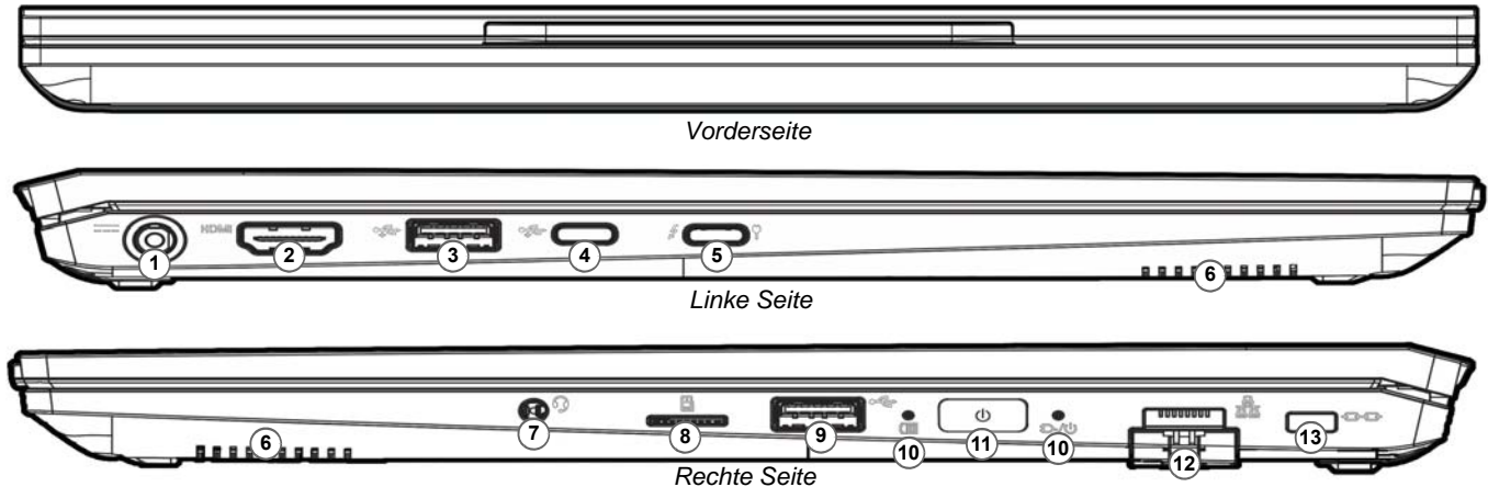
Abb. 4 - Ansicht von vorne, links und rechts (Modell A)
