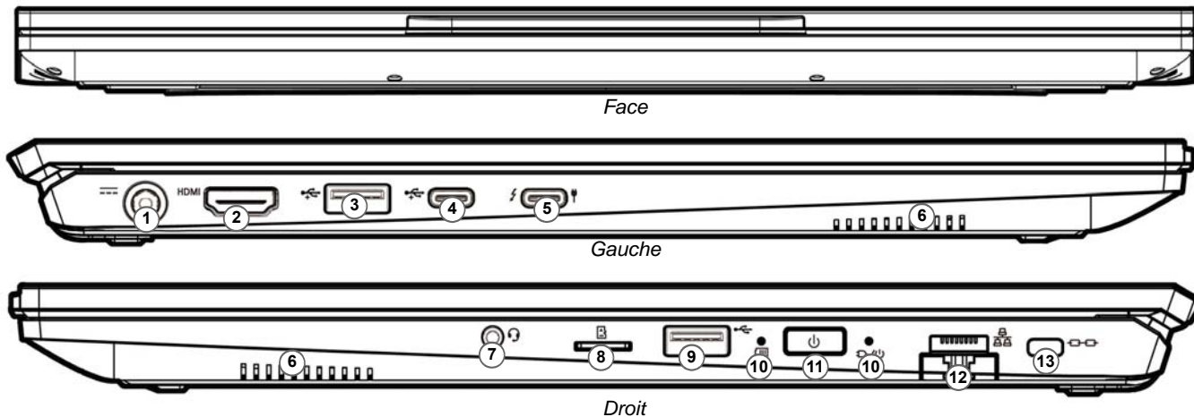
Figure 5 - Vues de face, gauche et droite (Modèle B)
