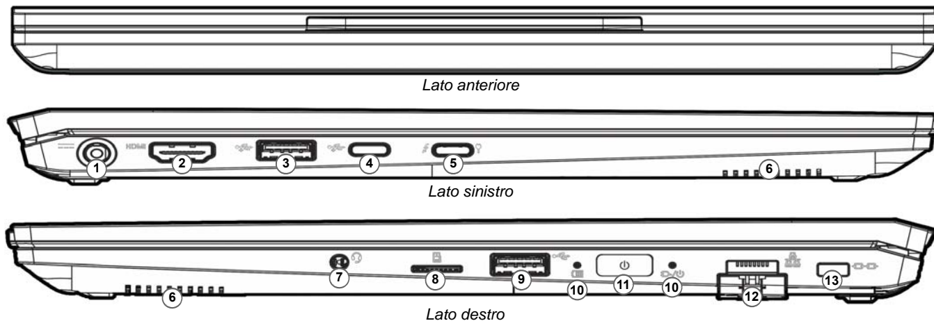
Figura 4 - Vista anteriore, sinistra e destra (Modello A)
