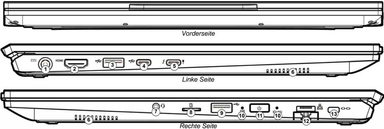
Abb. 5 - Ansicht von vorne, links und rechts (Modell B)
