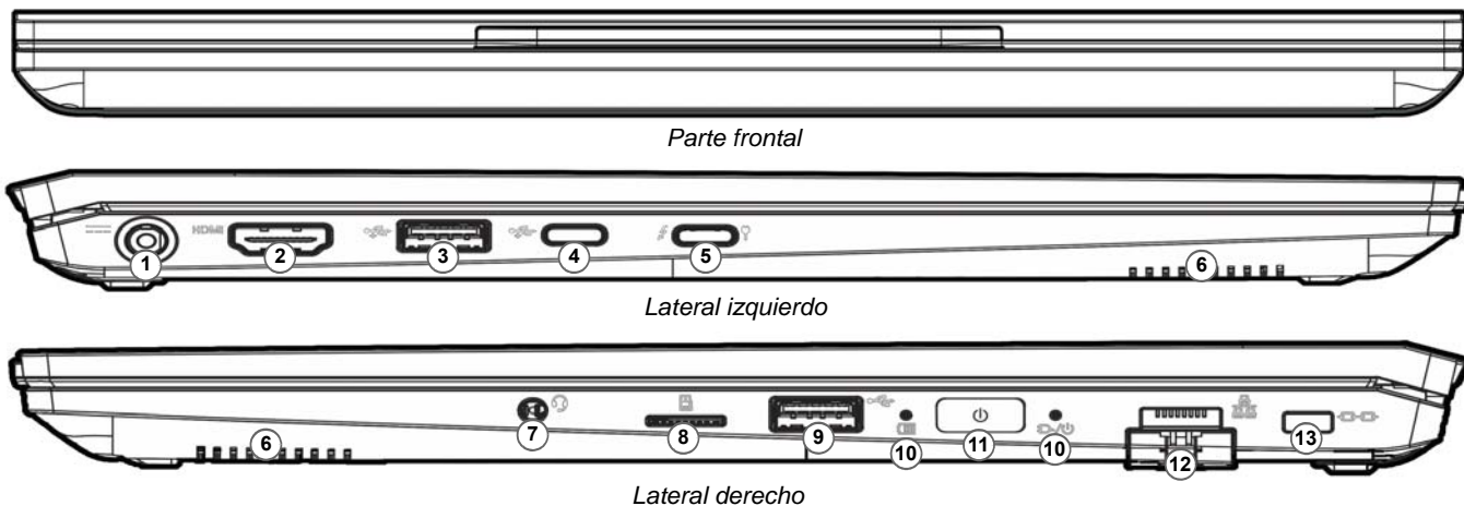
Figura 4 - Vistas frontal, izquierda y derecha (Modelo A)
