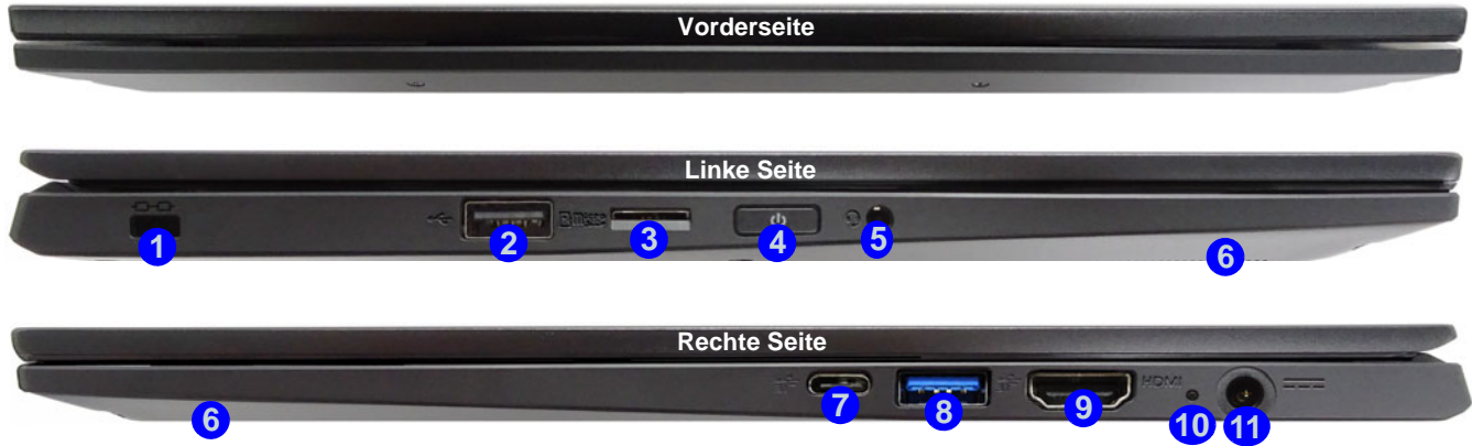
Abb. 7- Ansicht von vorne, links und rechts (Modell A)
