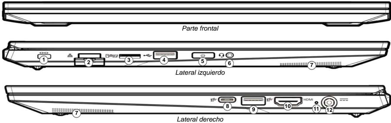
Figura 11 - Vistas frontal, izquierda y derecha (Modelo A)
