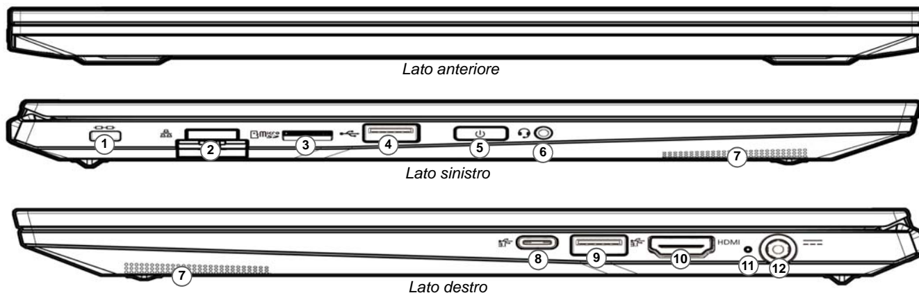
Figura 11 - Vista anteriore, sinistra e destra (Modello A)
