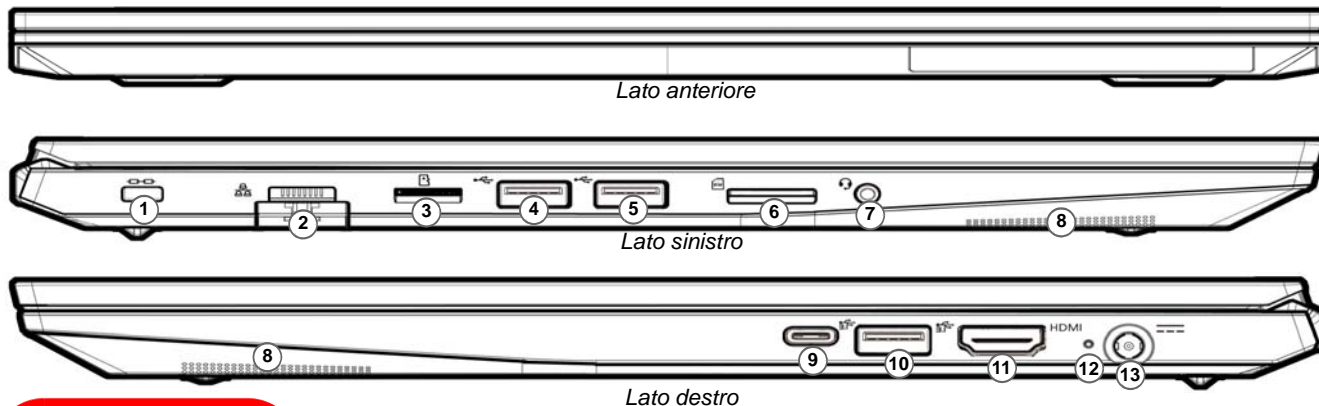
Figura 12 - Vista anteriore, sinistra e destra (Modello B)
