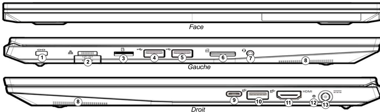
Figure 12 - Vues de face, gauche et droite (Modèle B)
