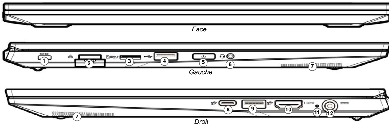
Figure 11 - Vues de face, gauche et droite (Modèle A)
