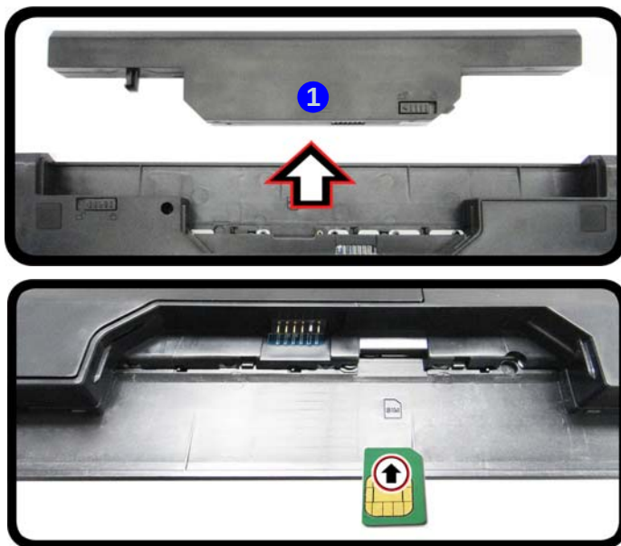
Figura 15 - Rimozione della batteria e inserimento della carta USIM
