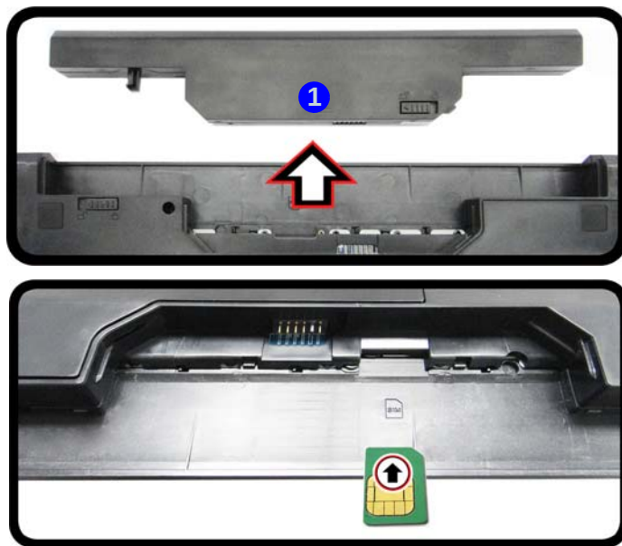
Figura 15 - Quitar la batería e insertar la tarjeta USIM
