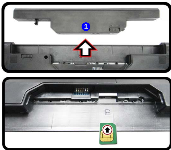
Figure 15 - Retirer la batterie et insérer la carte USIM
