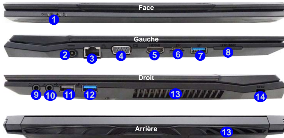
Figure 14 - Vues de face, gauche, droite et arrière (Modèle A)
