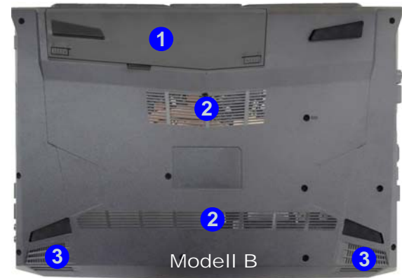
Abb. 17 Ansicht von unten
