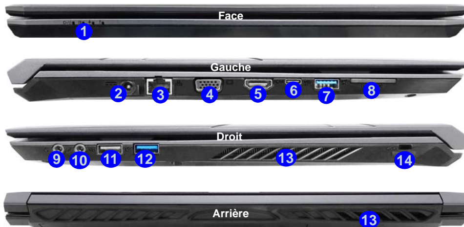
Figure 15 - Vues de face, gauche, droite et arrière (Modèle B)
