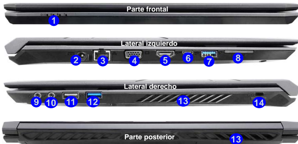
Figura 15 - Vistas frontal, izquierda, derecha y posterior (Modelo B)
