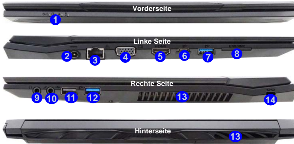
Abb. 14 - Ansicht von vorne, links, rechts und hinten (Modell A)
