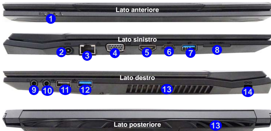
Figura 14 - Vista anteriore, sinistra, destra e posteriore (Modello A)
