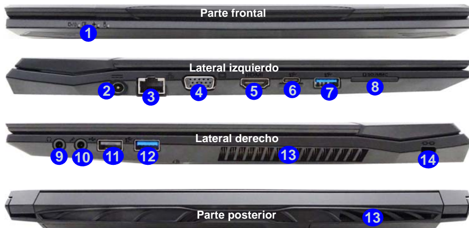
Figura 14 - Vistas frontal, izquierda, derecha y posterior (Modelo A)
