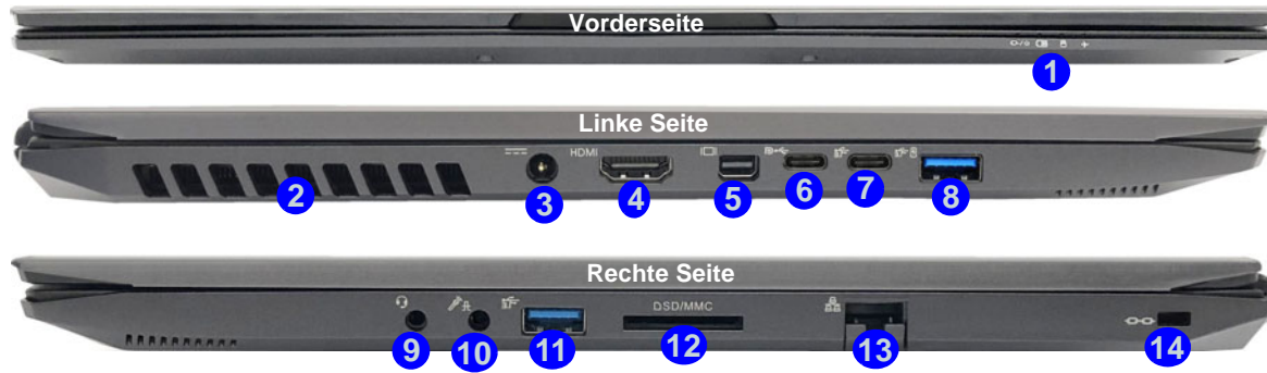
Abb. 5 - Ansicht von vorne, links und rechts (Modell C)
