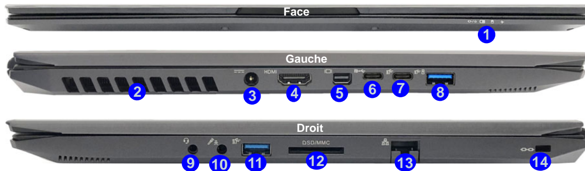
Figure 5 - Vues de face, gauche et droite (Modèle C)
