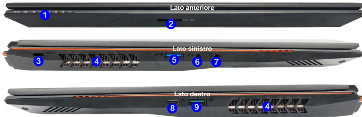
Figura 4 - Vista anteriore, sinistra e destra
