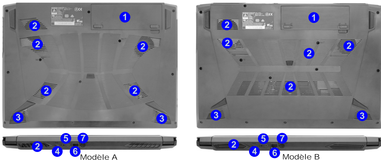
Figure 5 Vues de dessous et arrière
