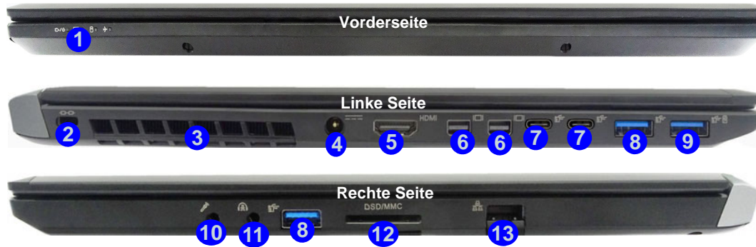
Abb. 5 - Ansicht von vorne, links und rechts
