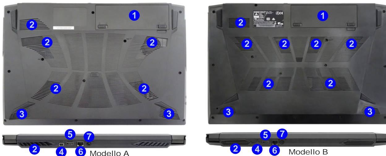
Figura 6 Vista inferiore e posteriore
