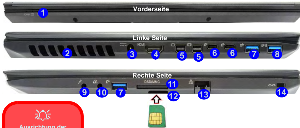
Abb. 5 - Ansicht von vorne, links und rechts (Modell A)
