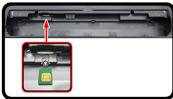
Figura 17 Quitar la batería e insertar la tarjeta USIM
