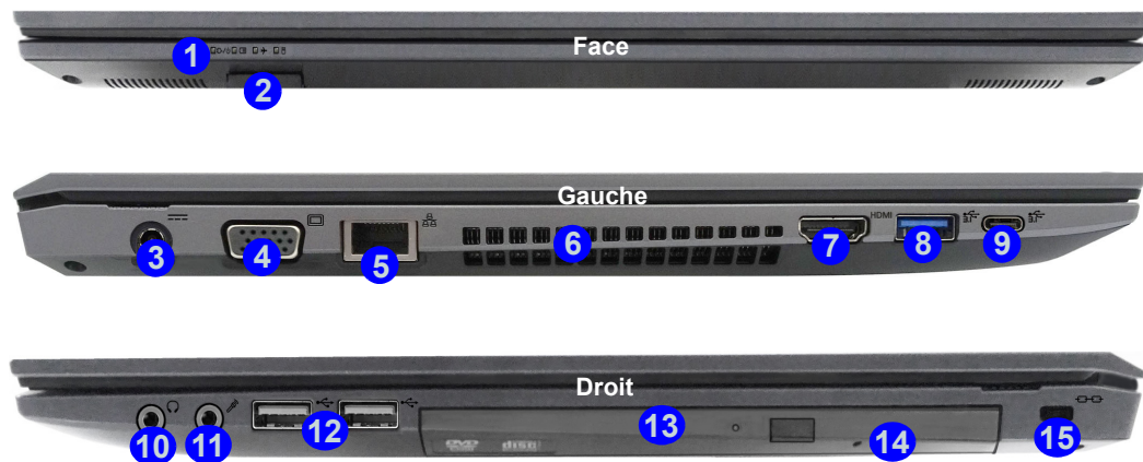
Figure 7 - Vues de face, gauche et droite (Modèle A)
