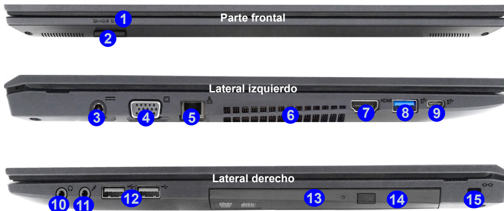
Figura 8 - Vistas frontal, izquierda y derecha (Modelo B)
