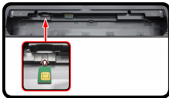
Figure 17 Retirer la batterie et insérer la carte USIM
