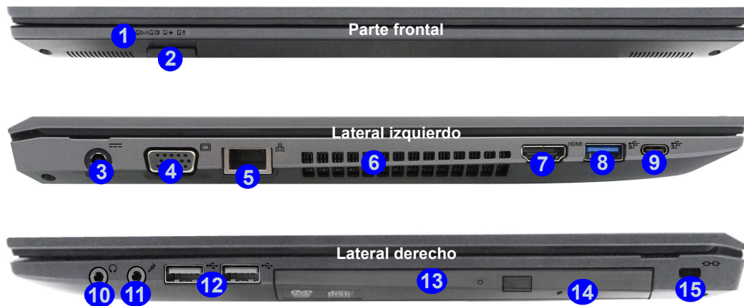
Figura 7 - Vistas frontal, izquierda y derecha (Modelo A)
