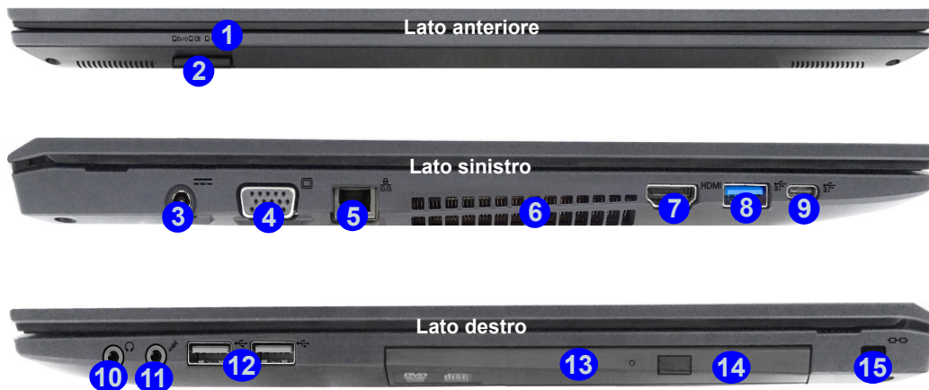
Figura 8 - Vista anteriore, sinistra e destra (Modello B)
