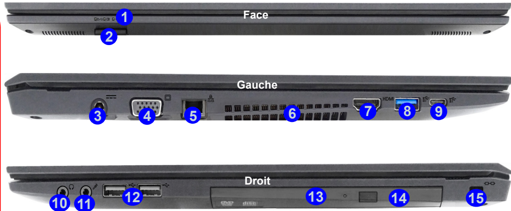
Figure 8 - Vues de face, gauche et droite (Modèle B)
