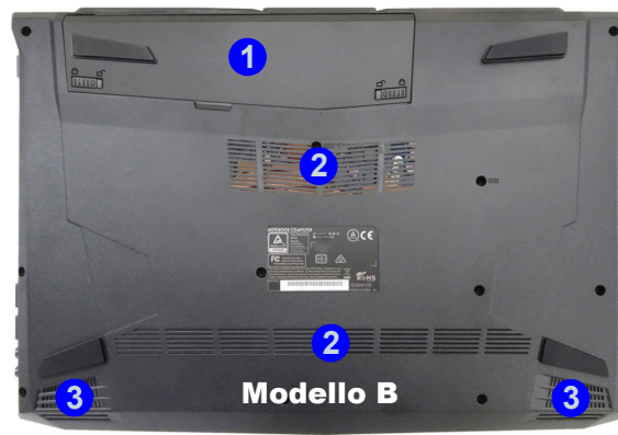
Figura 10 Vista inferiore
