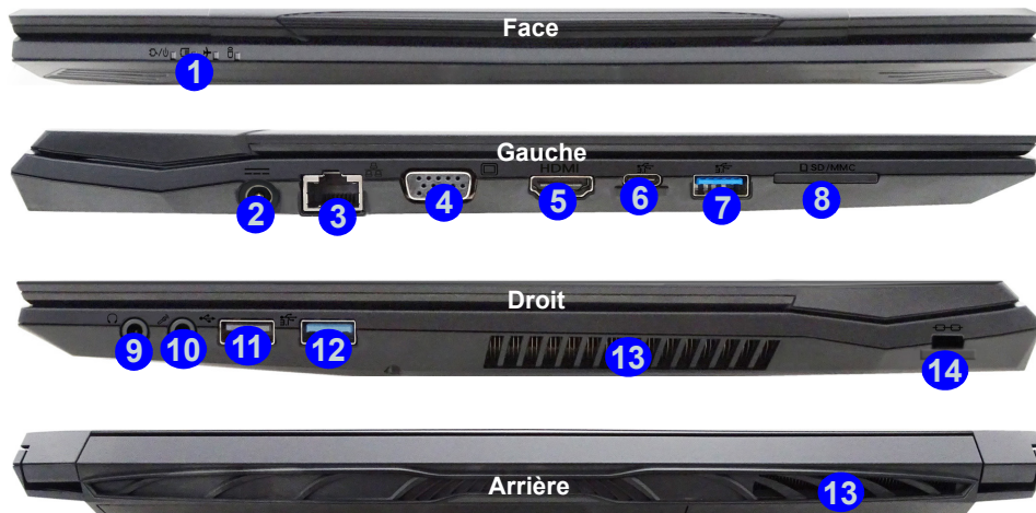
Figure 7 - Vues de face, gauche, droite et arrière (Modèle A)
