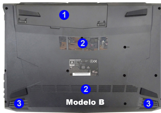
Figura 10 Vistas inferiores
