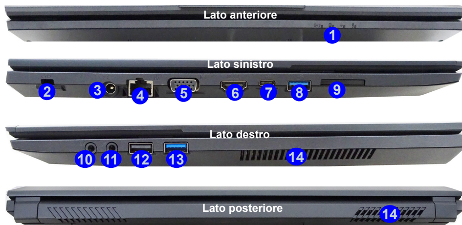
Figura 9 - Vista anteriore, sinistra, destra e posteriore (Modello C)
