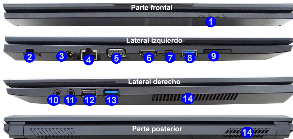
Figura 9 - Vistas frontal, izquierda, derecha y posterior (Modelo C)
