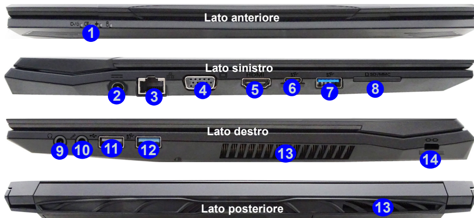
Figura 7 - Vista anteriore, sinistra, destra e posteriore (Modello A)
