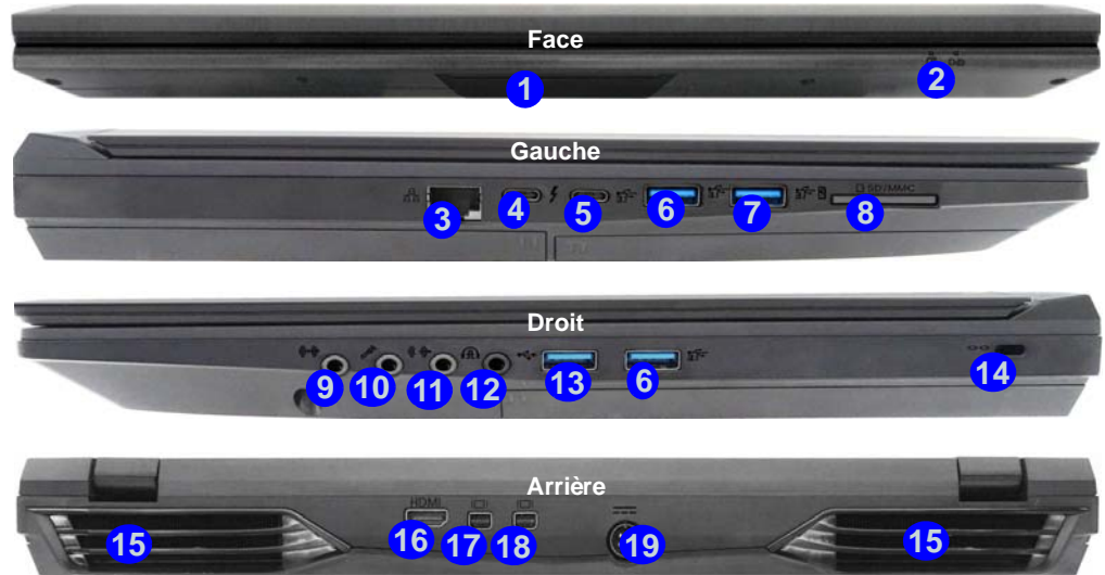
Figure 6 - Vues de face, gauche, droite et arrière (Modèles A & B)
