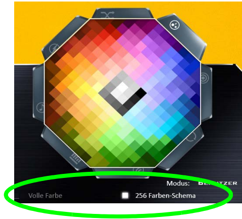
Abb. 24 - Farbmuster
