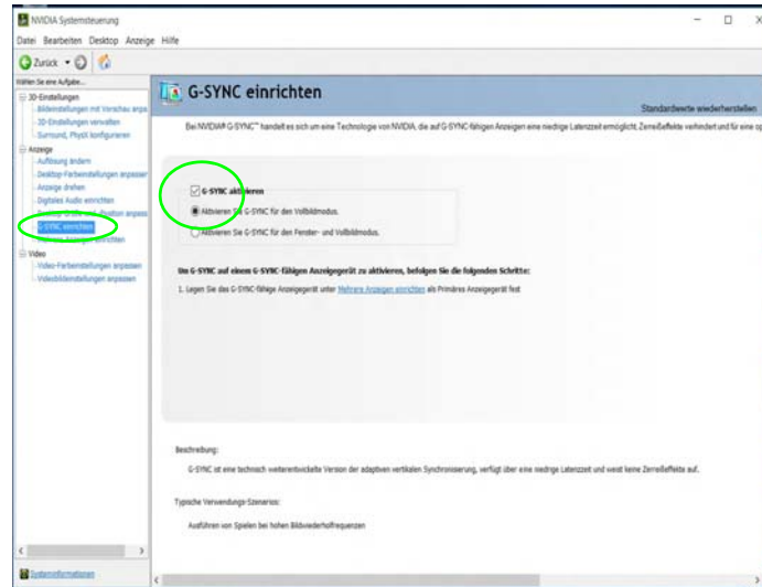
Abb. 29 - G-SYNC einrichten
