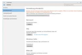
Abb. 34 Konten - Anmeldeoptionen
