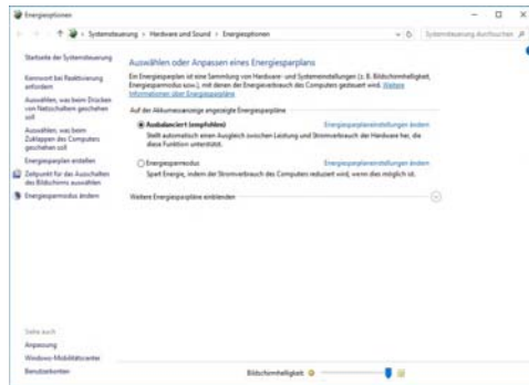
Abb. 30 - Energieoptionen
