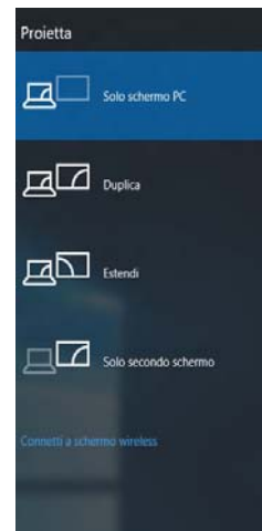
Figura 28 Proietta
