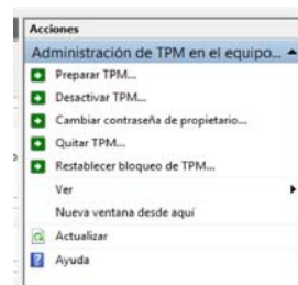
Figura 37 Menú Acciones
