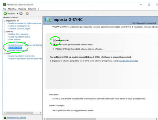
Figura 29 - Imposta G-SYNC
