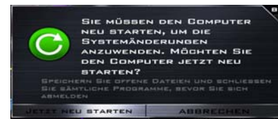
Abb. 13 - Speicher-Übertaktung
