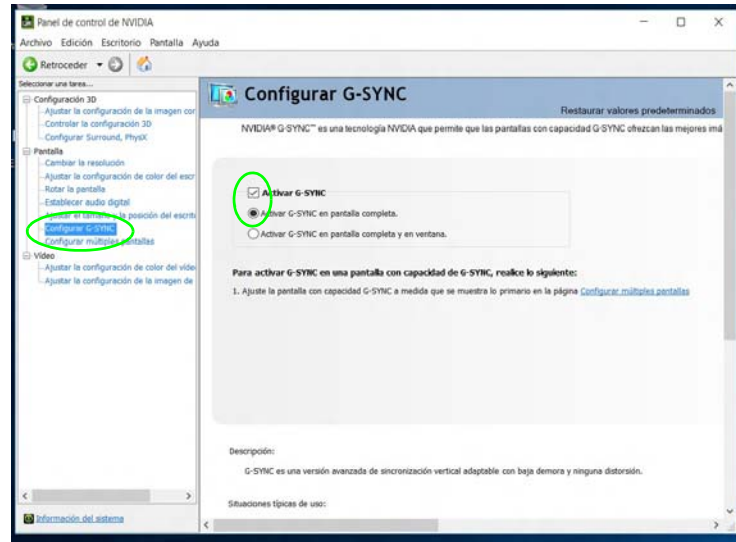
Figura 29 - Configurar G-SYNC
