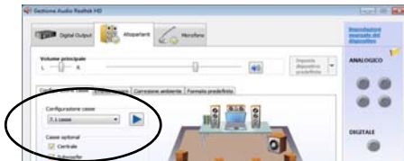
Figura 31 Configurazione casse
