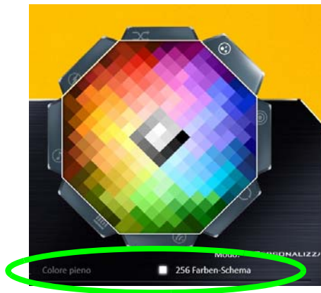
Figura 24 - Campione colore
