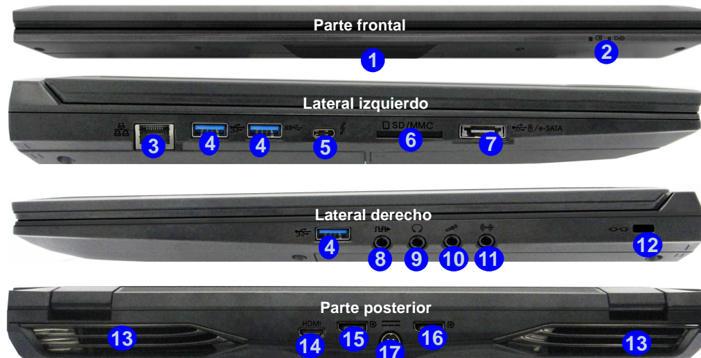
Figura 19 Vistas frontal, izquierda, derecha y posterior (Modelo B)
