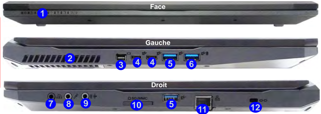
Figure 13 - Vues de face, gauche et droite (Modèle B)
