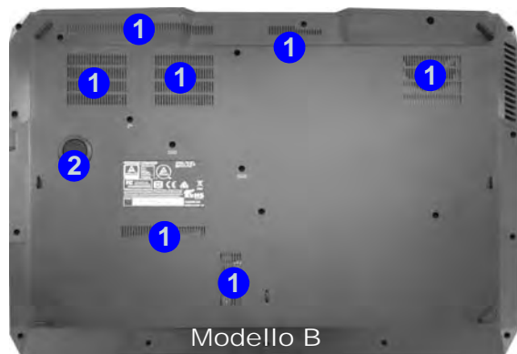
Figura 14 Vista inferiore e posteriore (Modelli A & B)
