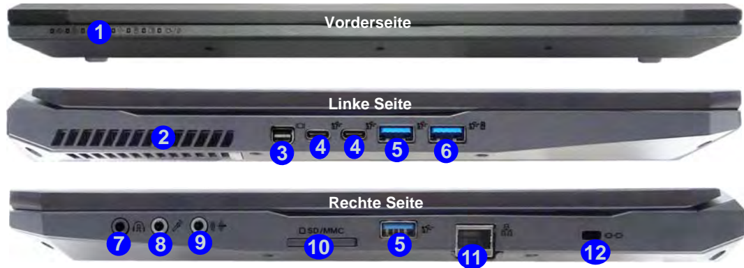
Abb. 13 - Ansicht von vorne, links und rechts (Modell B)
