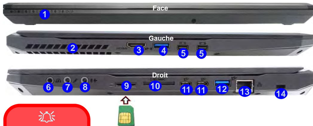
Figure 12 - Vues de face, gauche et droite (Modèle A - Design II)
