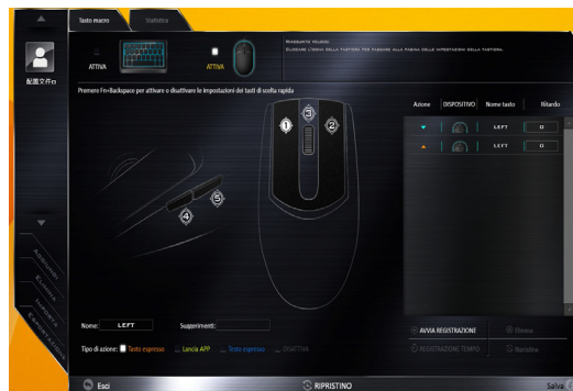
Figura 18 Configurazione mouse
