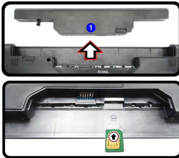
Figure 24 - Retirer la batterie et insérer la carte USIM
