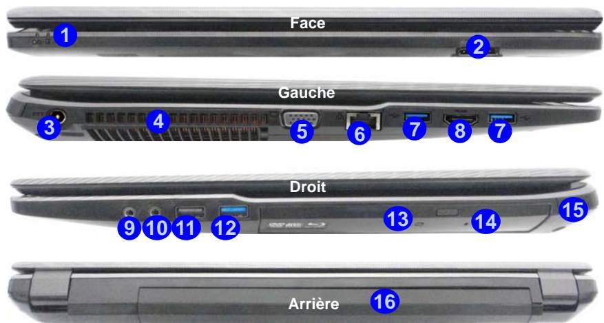
Figure 14 - Vues de face, gauche, droite et arrière (Modèle B)
