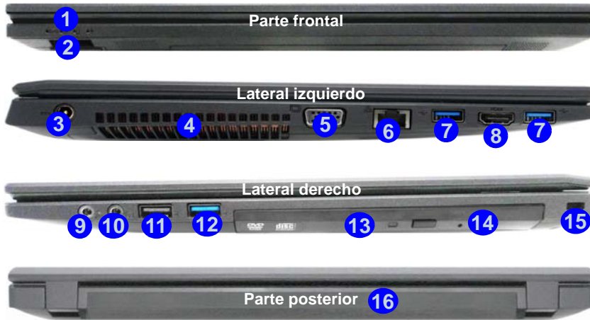
Figura 13 - Vistas frontal, izquierda, derecha y posterior (Modelo A)
