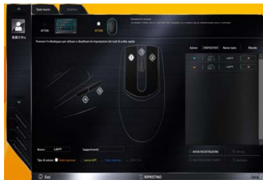
Figura 9 Configurazione mouse
