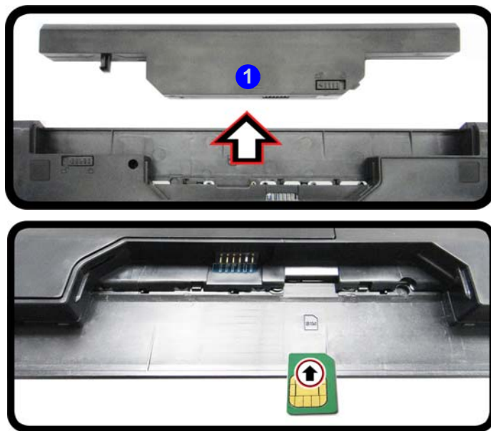
Figura 24 - Quitar la batería e insertar la tarjeta USIM
