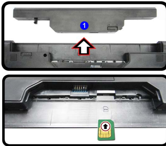
Abb. 24 - Herausnehmen des Akkus und einsetzen der USIM-Karte
