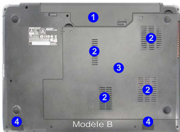
Figure 15 - Vues de dessous (Modèles A & B)
