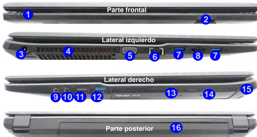
Figura 14 - Vistas frontal, izquierda, derecha y posterior (Modelo B)
