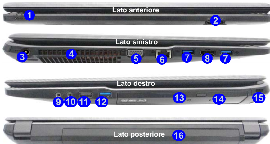
Figura 14 - Vista anteriore, sinistra, destra e posteriore (Modello B)
