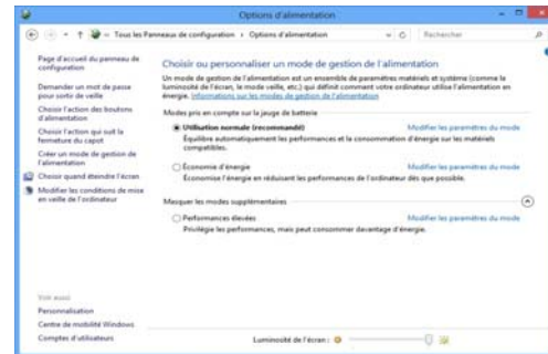
Figure 18 - Options d'alimentation
