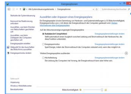
Abb. 18 - Energieoptionen
