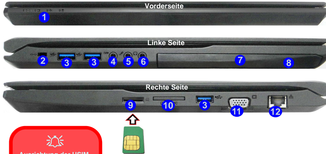
Abb. 13 - Ansicht von vorne, links und rechts (Modell B)
