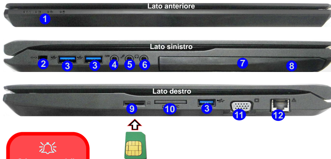
Figura 13 - Vista anteriore, sinistra e destra (Modello B)
