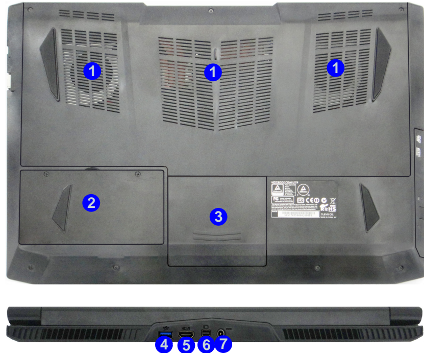
Abb. 16 - Ansicht von vorne, links und rechts (Modell C)
