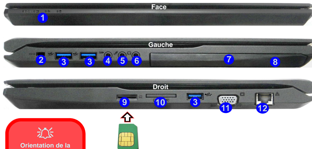
Figure 13 - Vues de face, gauche et droite (Modèle B)
