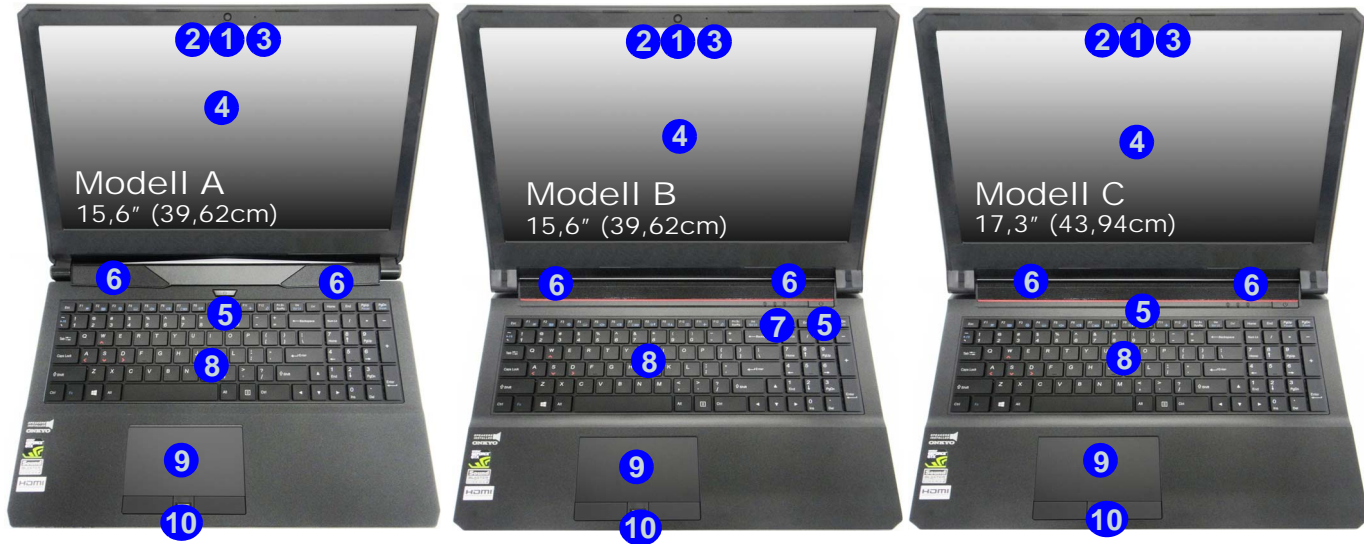
Abb. 2 - Ansicht von vorne mit geöffnetem LCD-Bildschirm (Modelle A, B & C)
