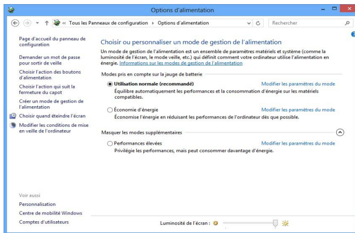
Figure 22 - Options d'alimentation
