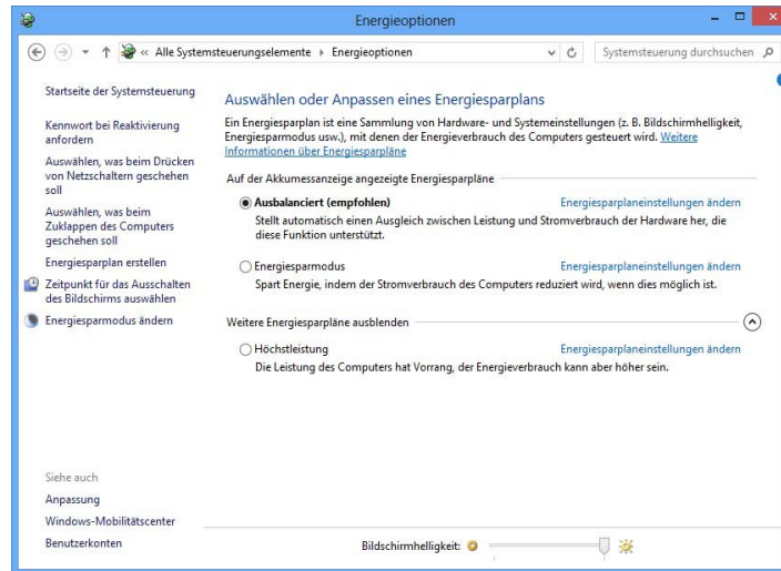
Abb. 22 - Energieoptionen
