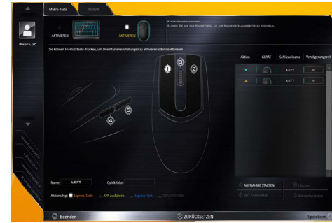
Abb. 8 - Mauskonfiguration
