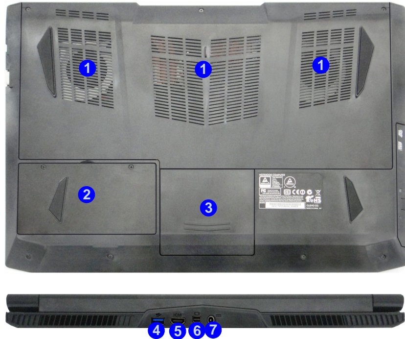
Figura 16 - Vistas inferior y posterior (Modelo C)
