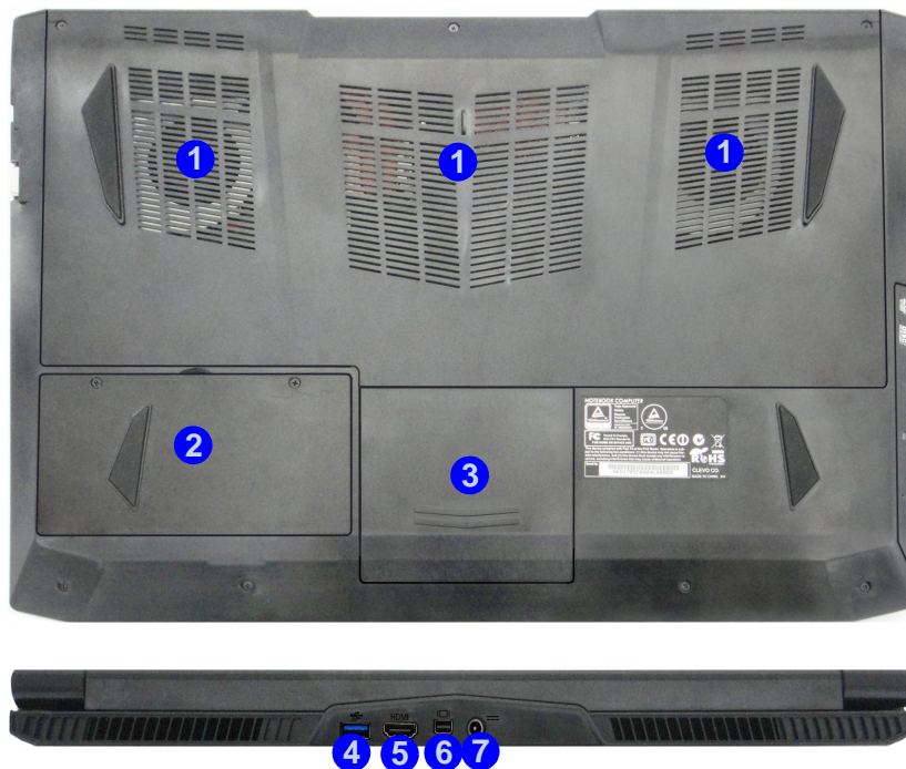
Figure 16 - Vues de dessous et arrière (Modèle C)
