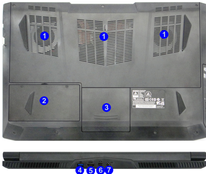
Figura 16 - Vista inferiore e posteriore (Modello C)
