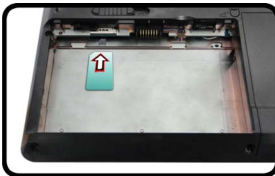
Figure 19 - Retirer la batterie et insérer la carte USIM
