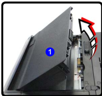
Figura 18 - Rimozione della batteria e inserimento della carta USIM
