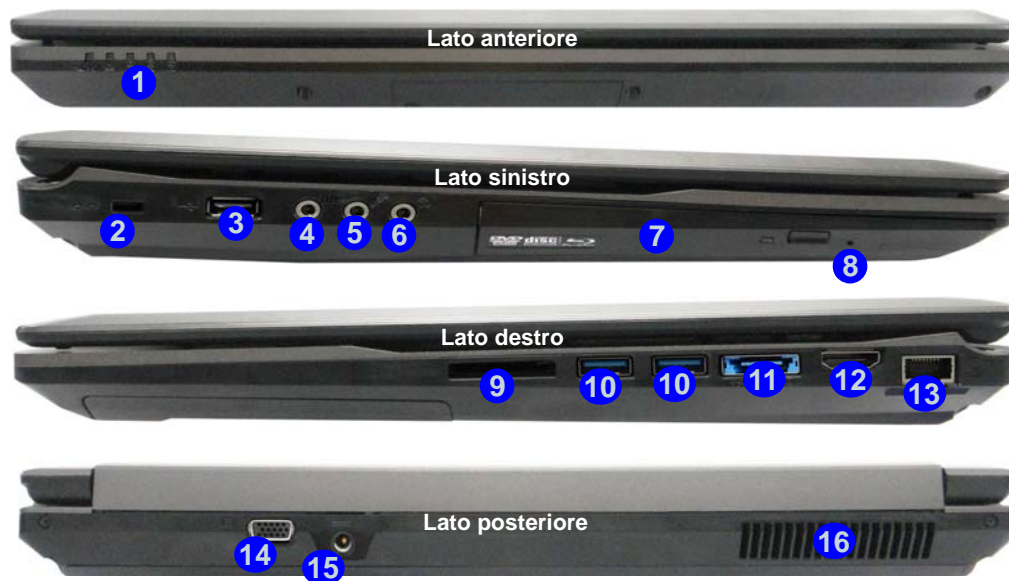
Figura 9 Vista anteriore, sinistra, destra e posteriore (Mo- delli A & C)
