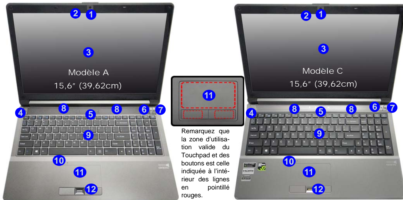
Figure 5 - Vue de face avec l'écran LCD ouvert (Modèles A & C)
