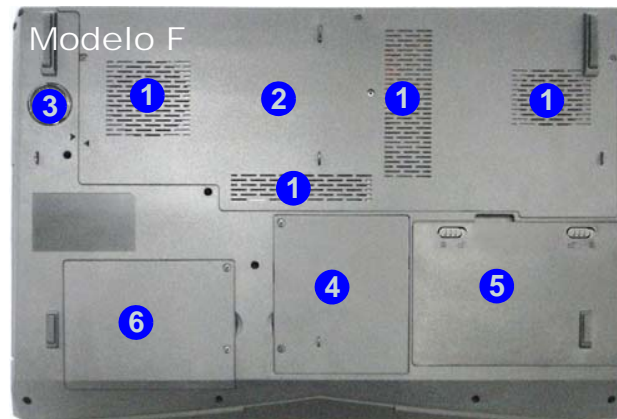
Figura 16 Vista inferior (Modelos E & F)
