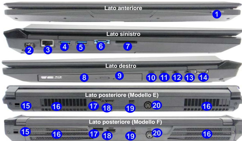
Figura 14 - Vista anteriore, sinistra, destra e posteriore (Modelli E & F)
