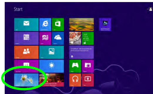
Abb. 7 Startbildschirm
