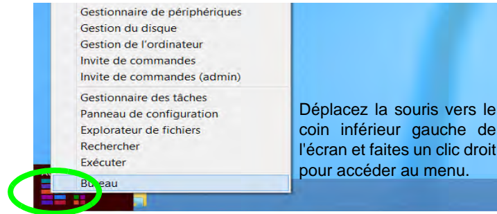
Figure 6 Menu contextuel
