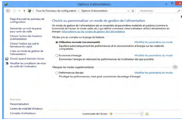
Figure 11 - Options d'alimentation
