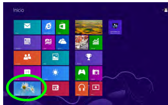
Figura 7 Pantalla Inicio
