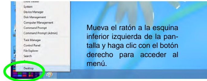
Figura 6 Menú contextual
