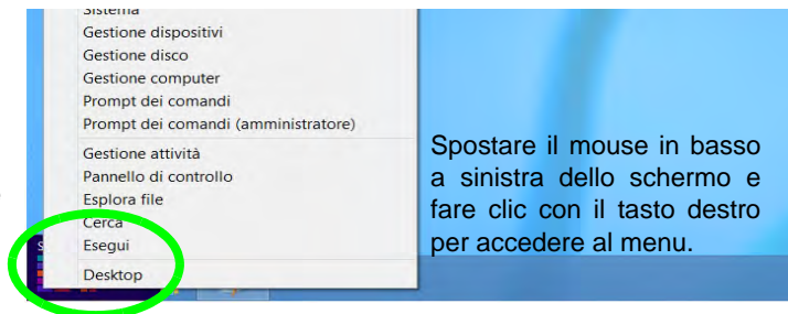
Figura 6 Menu contestuale
