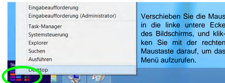
Abb. 6 Kontextmenü
