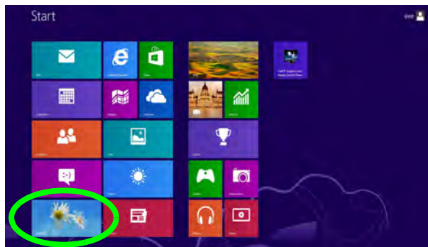
Figura 7 Schermata Start
