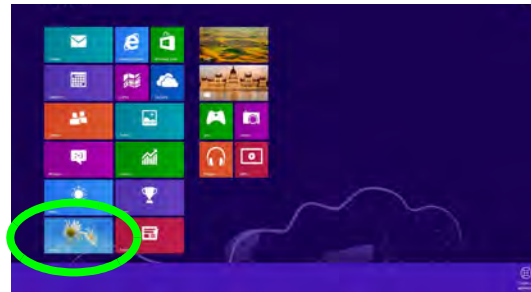
Figure 7 Écran d'accueil
