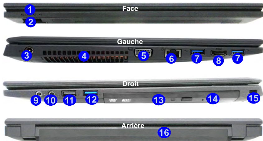
Figure 14 - Vues de face, gauche, droite et arrière (Modèle A)
