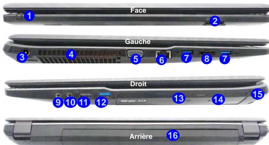
Figure 15 - Vues de face, gauche, droite et arrière (Modèle B)
