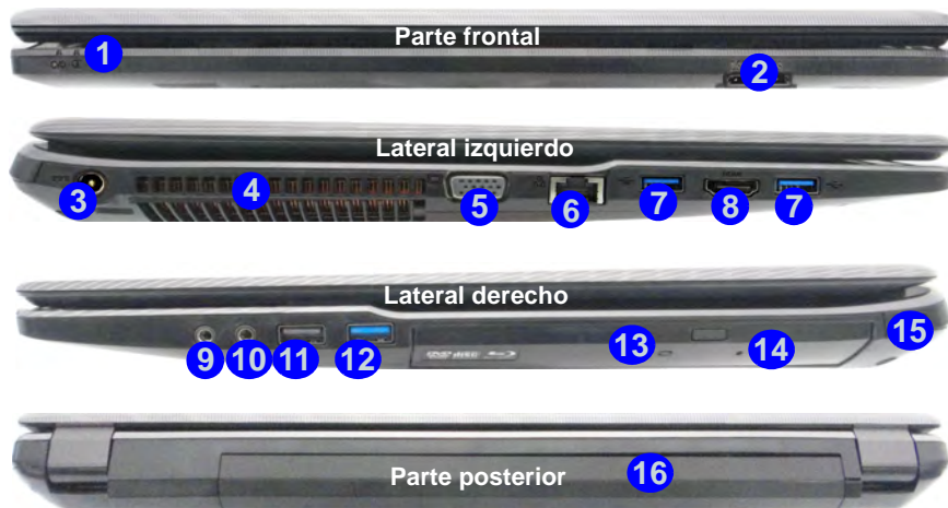
Figura 15 - Vistas frontal, izquierda, derecha y posterior (Modelo B)
