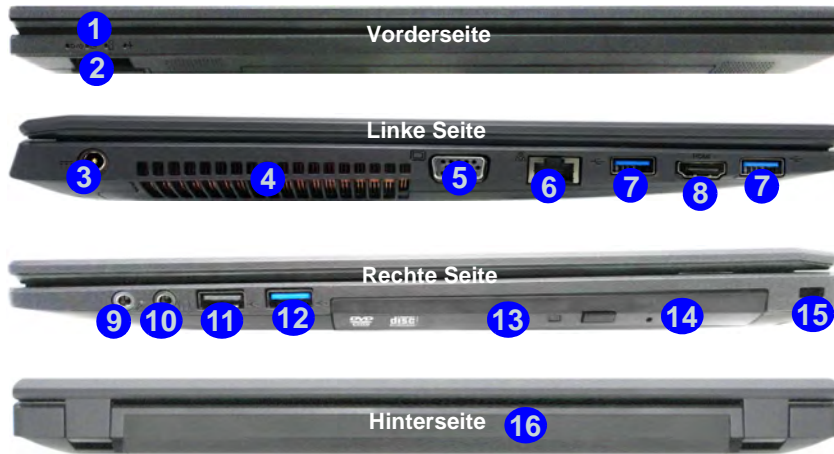
Abb. 14 - Ansicht von vorne, links, rechts und hinten (Modell A)
