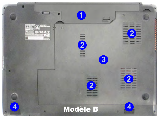
Figure 16 - Vues de dessous (Modèles A & B)
