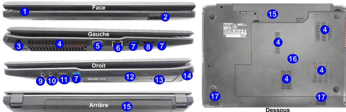
Figure 15 - Vues de face, gauche, droite, arrière et dessous (Modèle B)
