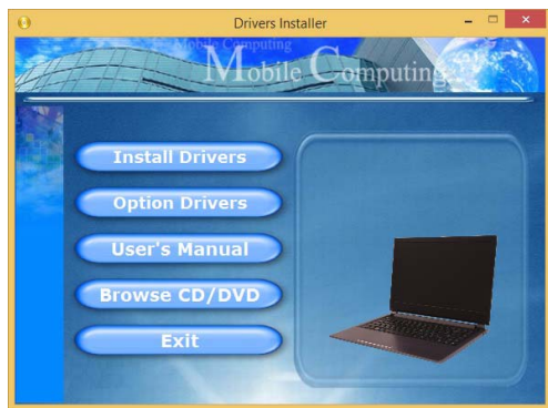
Figura 20 - Installazione driver
