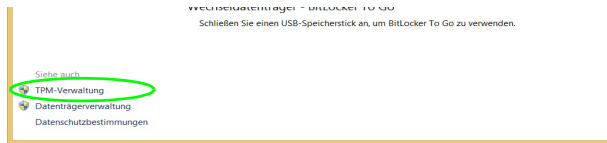
Abb. 21 - BitLocker-Laufwerkverschlüsselung (TPM-Verwaltung)
