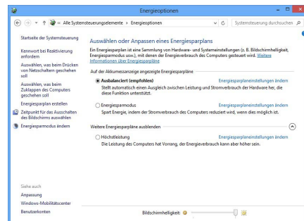
Abb. 18 - Energieoptionen
