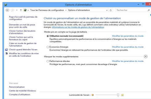
Figure 18 - Options d'alimentation
