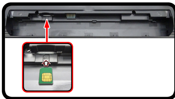
Figura 15 Quitar la batería e insertar la tarjeta USIM
