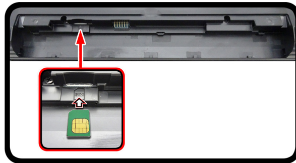
Figura 15 Rimozione della batteria e inserimento della carta USIM
