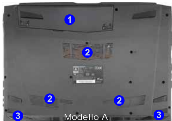
Figura 19 Vista inferiore
