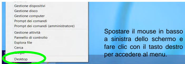
Figura 6 Menu contestuale
