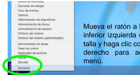
Figura 6 Menú contextual
