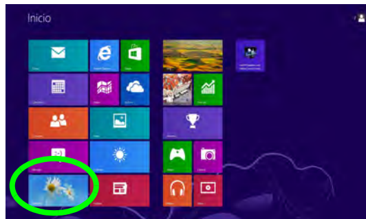
Figura 7 Pantalla Inicio
